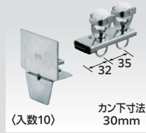
D40片マグネットランナー(片開)ステーションランナータイプ
